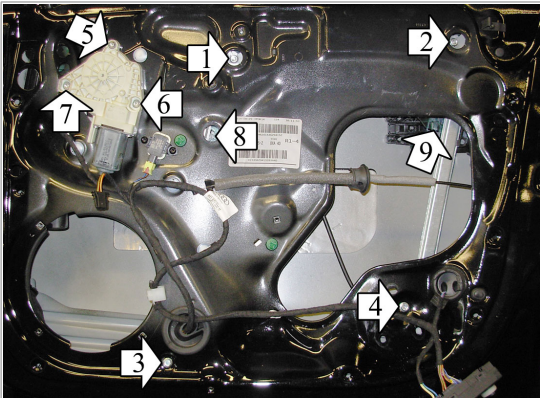
A POWER WINDOW RIGHT ALZACRISTALLI ELETTRICO DX
