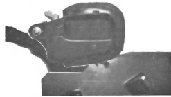
RE ASSEMBLY OF INTERNAL DOOR RELEASE HANDLE. MONTAGE DE LA COMMANDE POUR L'OUVERTURE DE LA PORTE. MONTAGE DES TÜRÖFFNUNGSSANTREIS. MONTAJE TIRADOR APERTURA PUERTA. MONTAGGIO COMANDO APERTURA PORTA.
