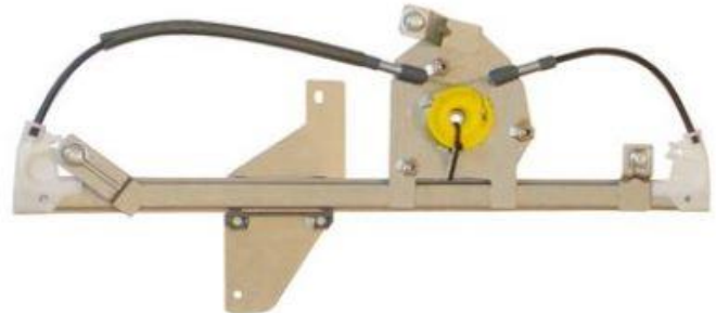
ALZACRISTALLO ELETTRICO SINISTRO POWER WINDOW LEFT
