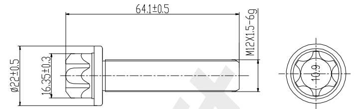
Bolt 3PCS DACRO
