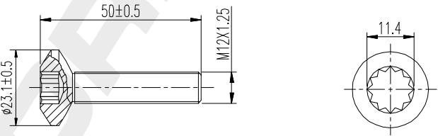
Bolt 163-C-006 4PCS DACRO
